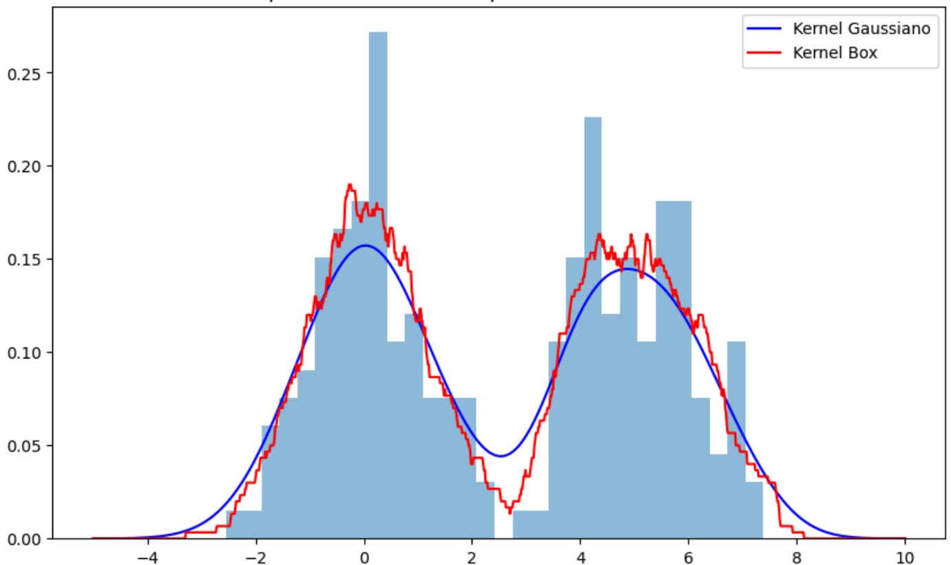
Comparación de suavizado por kernel: Gaussiano vs. Box
